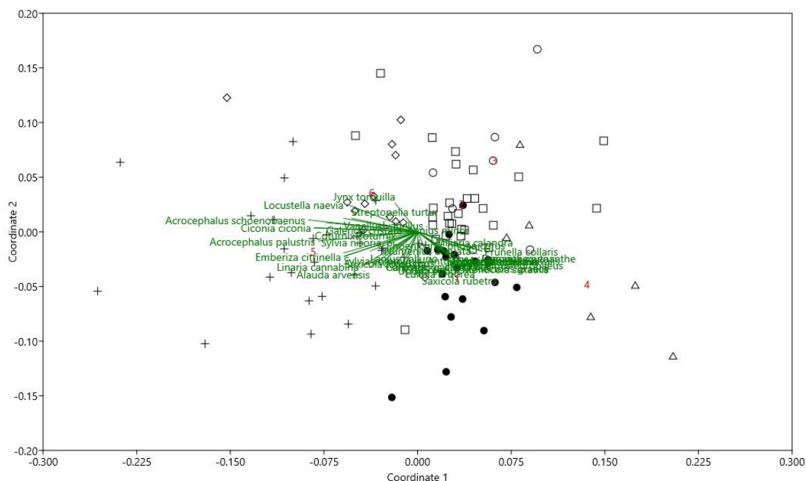
Slika 8. NMDS ordinacija Natura območij s pasivno projiciranimi vrstami ptic. Območja so razporejena v skupine glede na klasifikacijo, rdeče številke predstavljajo centroe klastrov. Uporabili smo evklidsko razdaljo.
